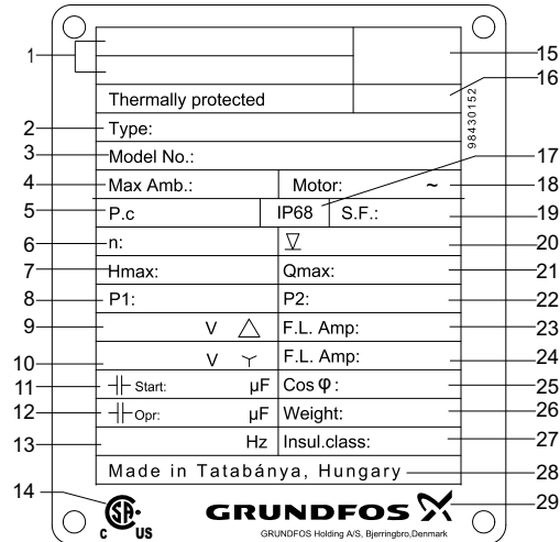
Fig. 2 SEG nameplate
